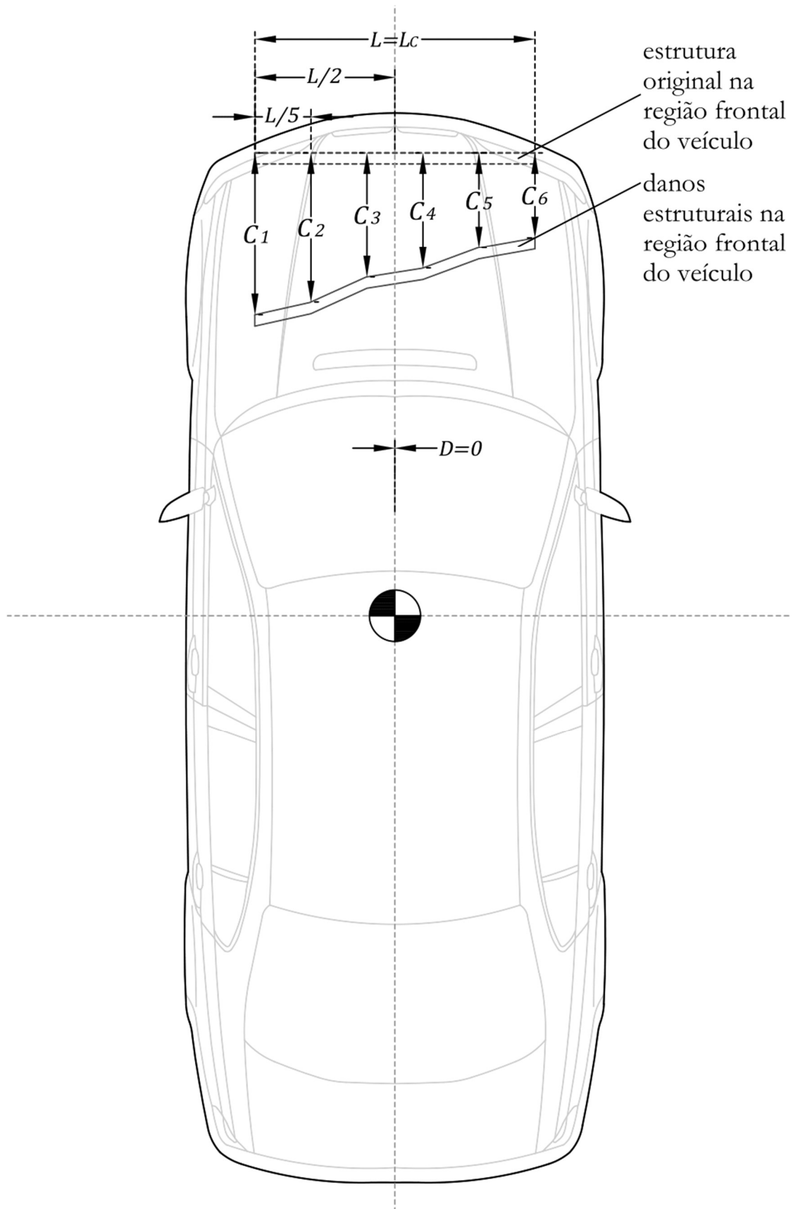
Figura 4.52 Protocolo utilizado para realizar a medição das cotas reais do perfil de deformação frontal.
