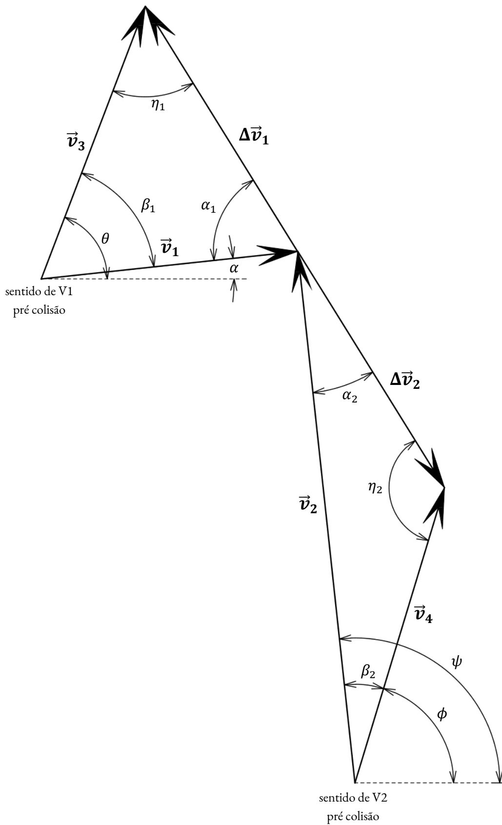
Figura 3.10 Análise vetorial entre os vetores velocidade imediatamente antes, durante e após a colisão para ambos veículos. Os ângulos \eta são explicados no Capítulo 4.
