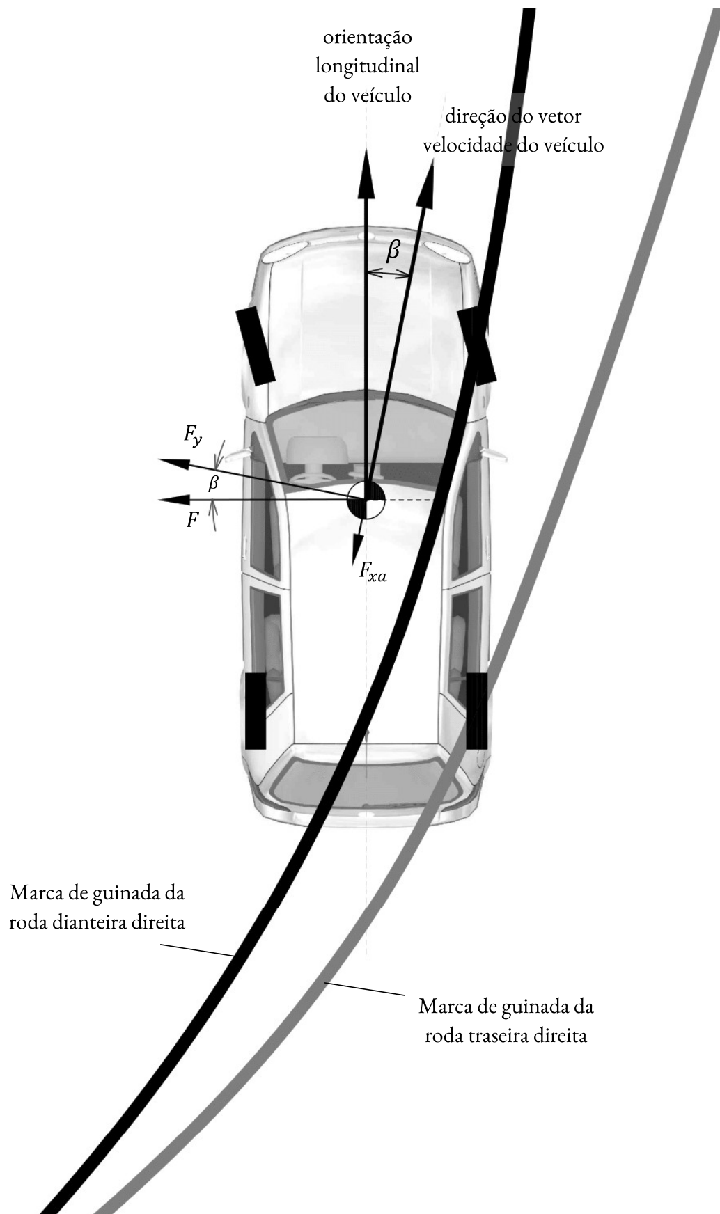
Figura 2.60 Análise de forças no veículo realizando uma manobra curva.
